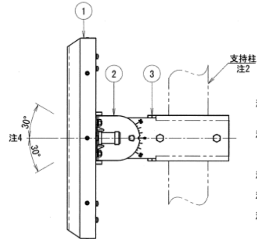
取付タイプ1(V偏波) 注1
