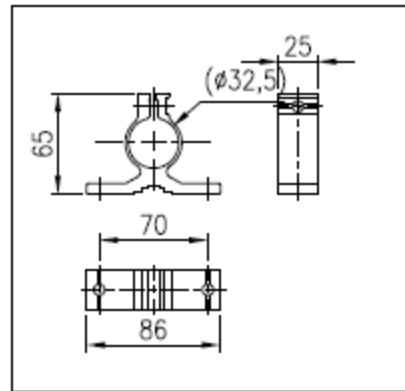
取付金具 (アンテナ1本につき2個使用)
