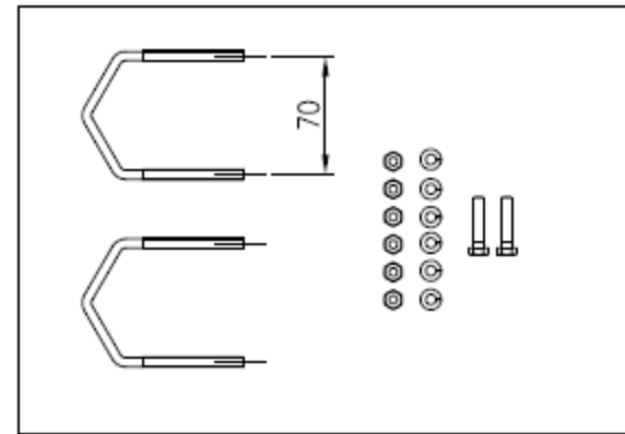
角U字ボルト 2本 M6 スプリングワッシャー 6枚 M6 六角ナット 6個 M6 x 30 六角ボルト 2本
