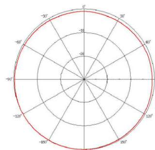
【1.5GHz帯水平面内】
