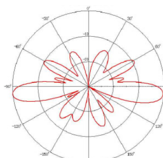
【1.7GHz帯垂直面内】
