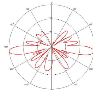
【2.0GHz帯垂直面内】
