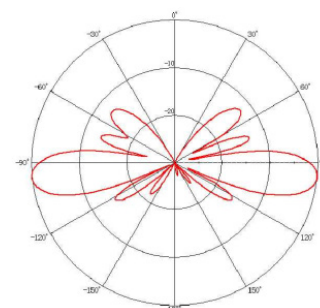
【1.5GHz帯垂直面内】
