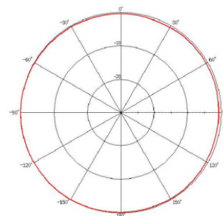
【2.0GHz帯水平面内】
