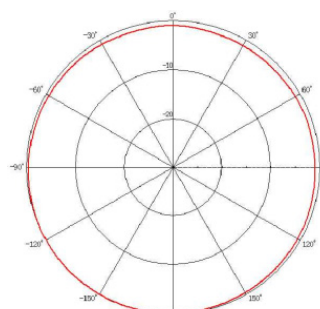
【1.7GHz帯水平面内】
