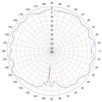
1695-2700MHz
