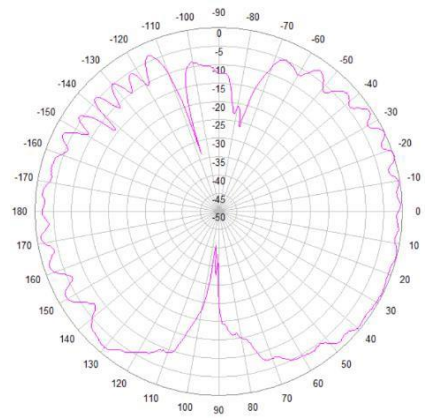
4900-6000MHz
