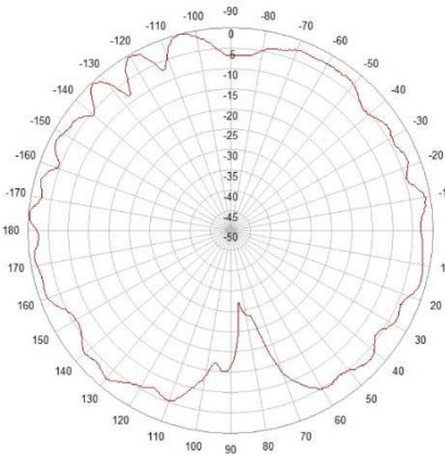
3300-3800MHz
