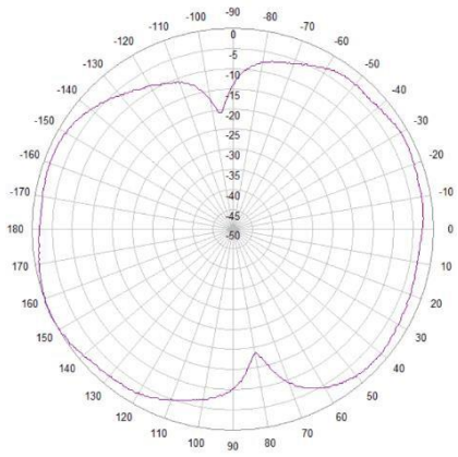
1695-2700MHz 6000MHz
